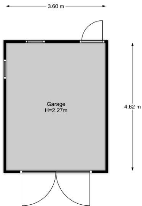
Begane grond, Broekhuizenstraat 11A te Terschuur De plattegronden zijn geschikt voor promotionele doeleinden. Er kunnen geen rechten aan ontleend worden. © Topr.nl
